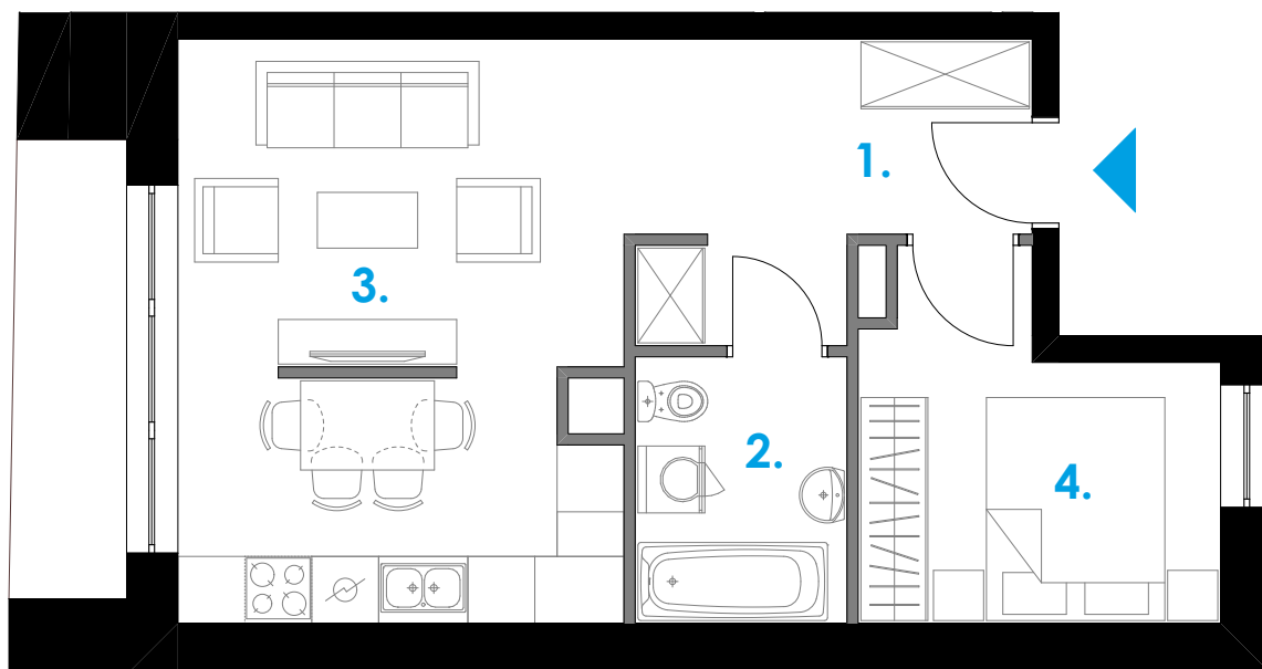
RZUT MIESZKANIA SKALA: 1:75
