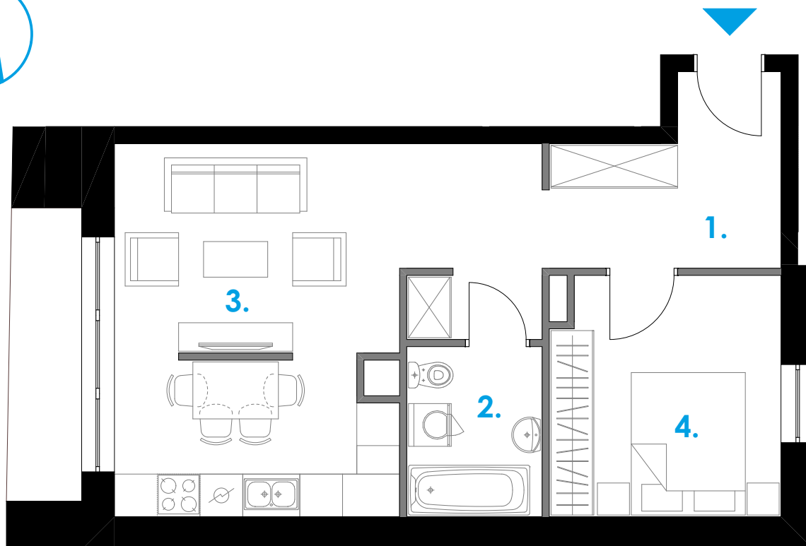
RZUT MIESZKANIA SKALA: 1:75
